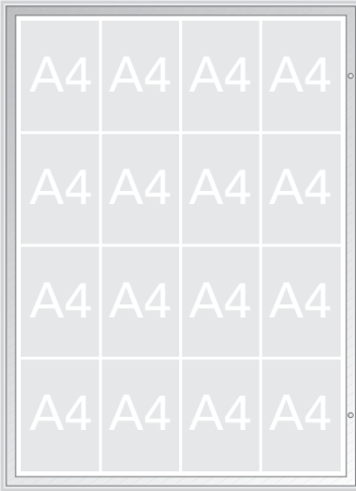
16 x A4 (Portrait) or A0 Exterior size (mm) 1350 x 1000 Visual area (mm) 1230 x 880
